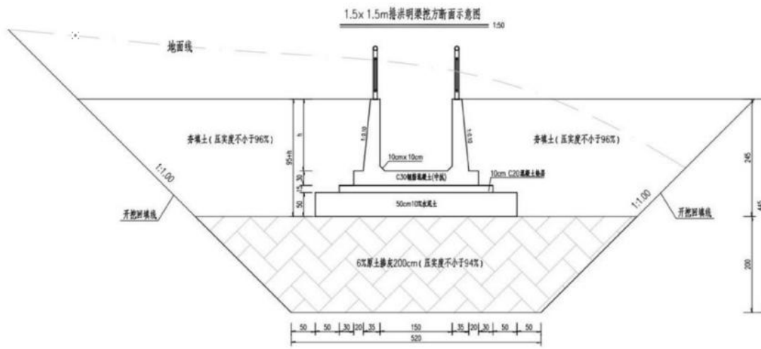
1.5×1.5m 排洪明渠挖方断面示意图
